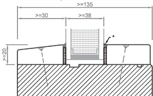
Abb. 2: Senkkopf-Holzschraube mit Vorlegeband*
